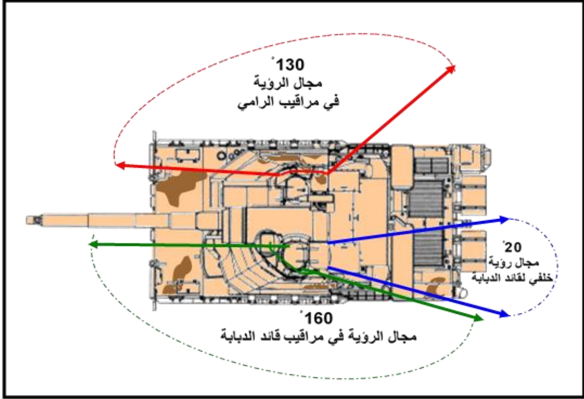
الشكل (1) مجال الرؤية بواسطة مراقيب قائد الدبابة والرامي
